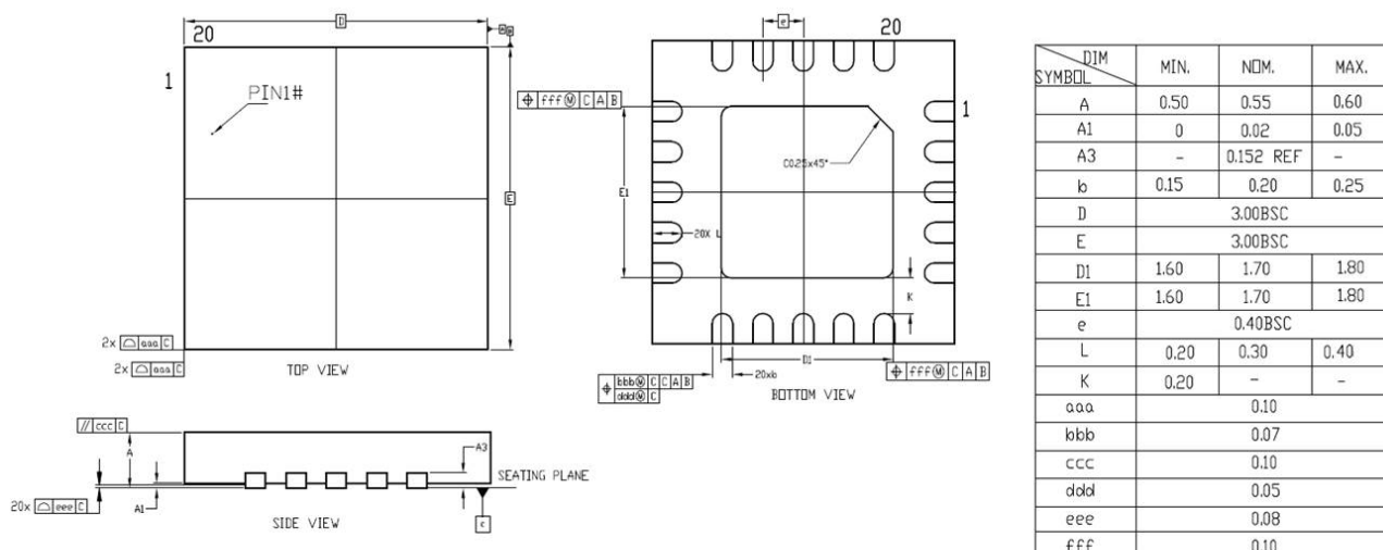
图 5-1: QFN20 封装图
