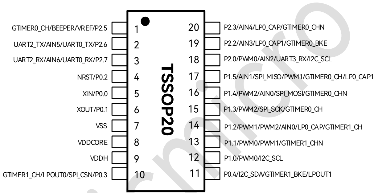
图 3-1: TSSOP20 封装管脚分布图
