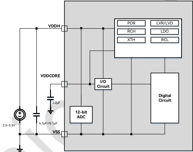
图 4-1：供电方案图
