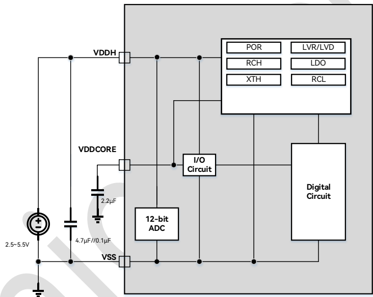
图 4-1：供电方案图
