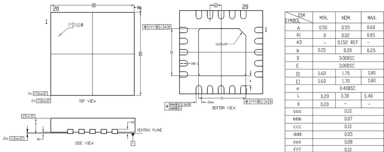
图 5-1: QFN20 封装图
