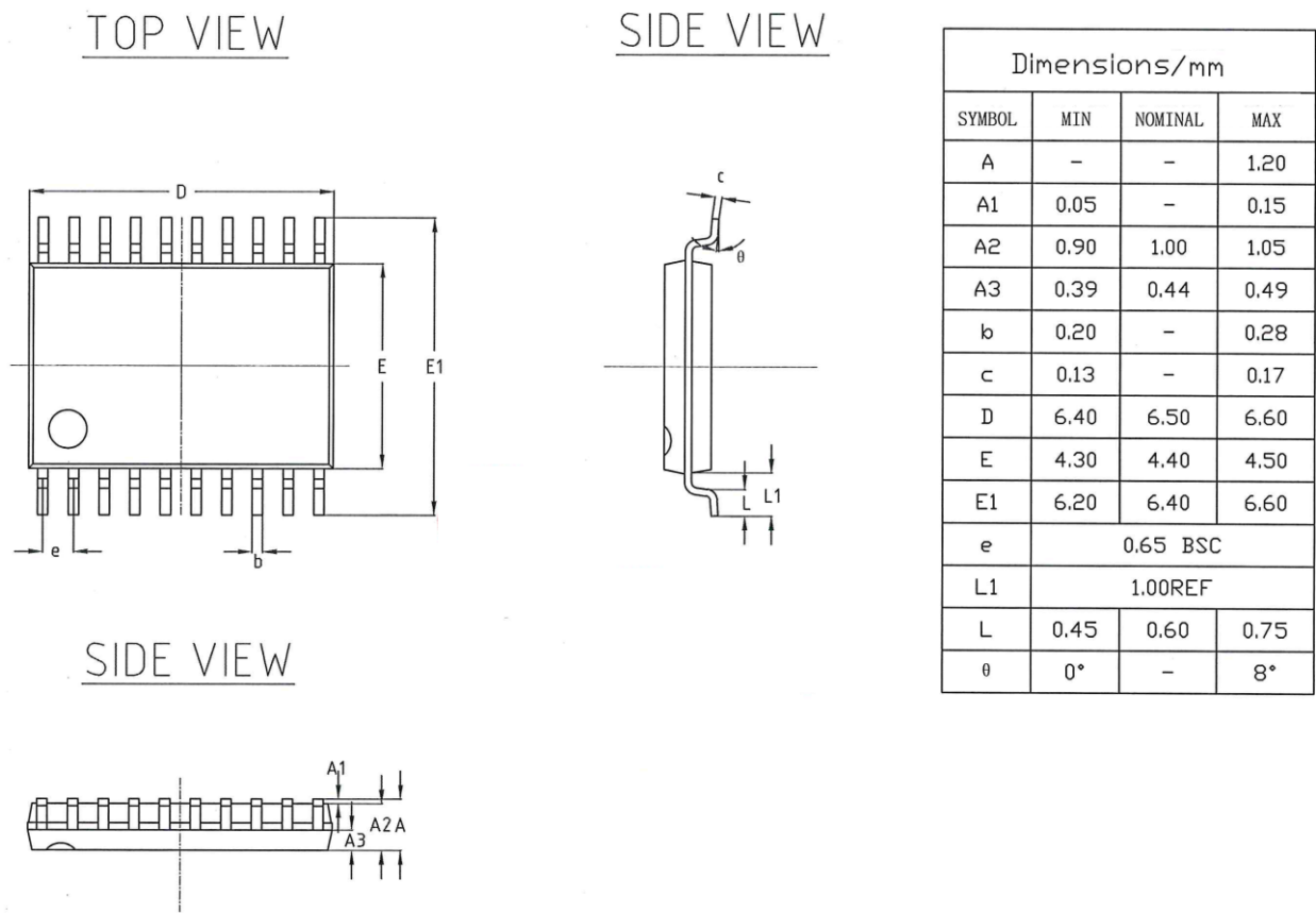
图 5-2: TSSOP20 封装图
