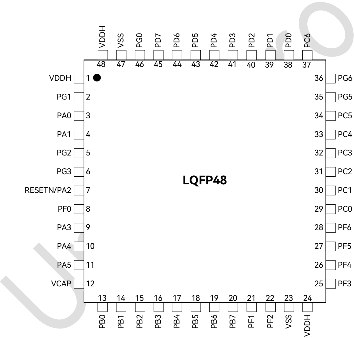
图 3-1：封装管脚分布图
