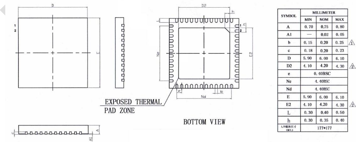
图 5-2: QFN48 封装图
