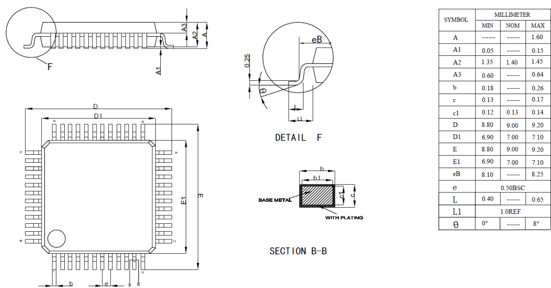
图 5-1: LQFP48 封装图
