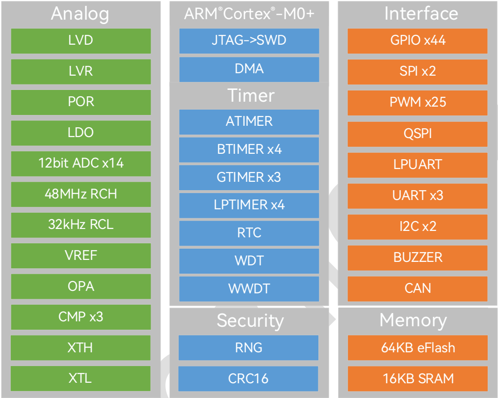
图 2-1：功能框图
