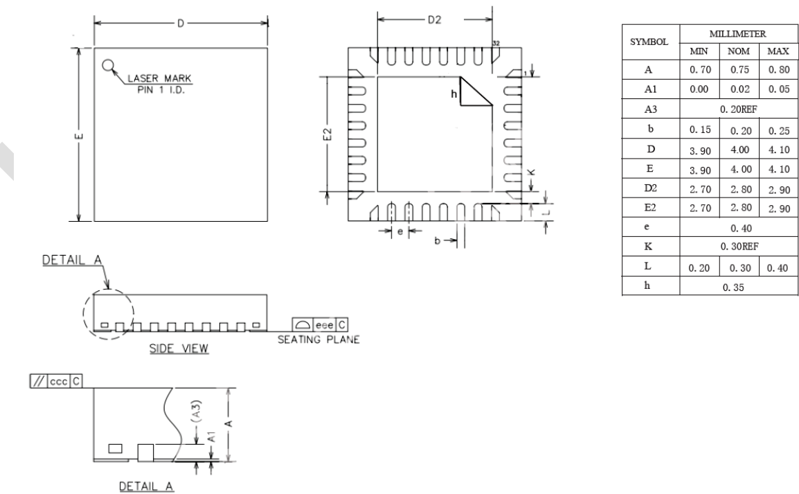
图 5-4: QFN32 封装图
